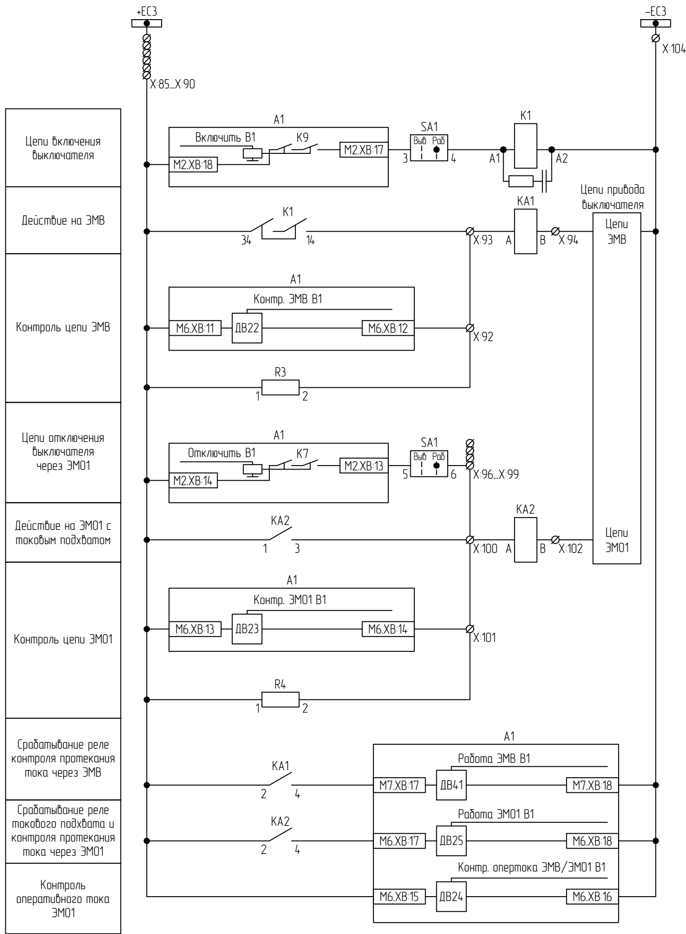
Цепи ЭМВ и ЭМ01
