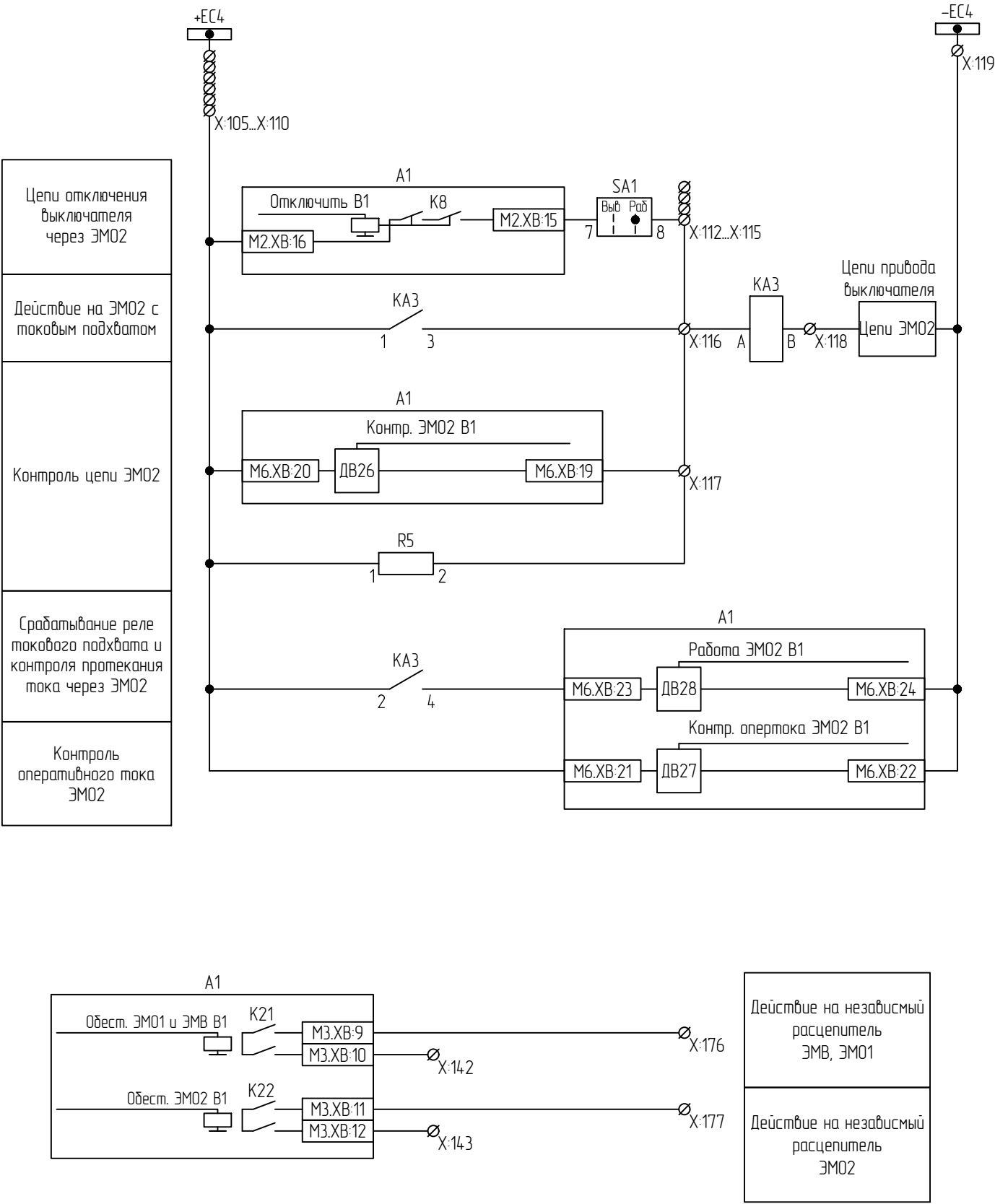
Цепи ЭМ02
